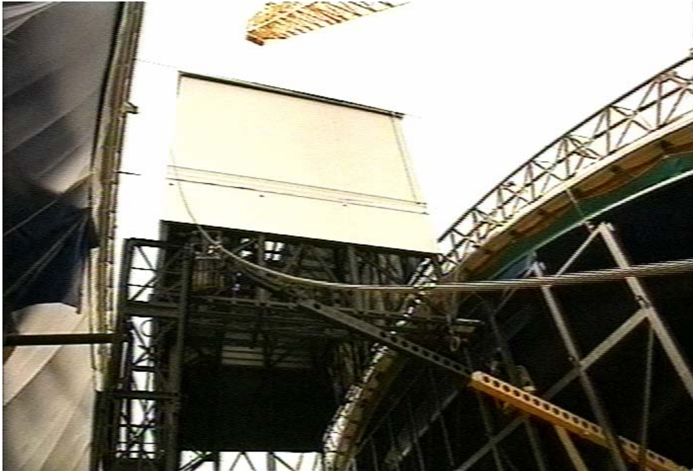
Sommer 2001: Einsatz des Bühnenturms mit Kran
